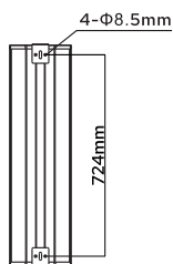
支架安装孔位
